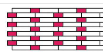
Цепная кладка
