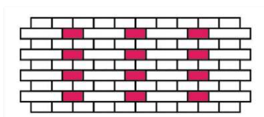
Голландская кладка
