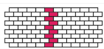
Тычковая кладка
