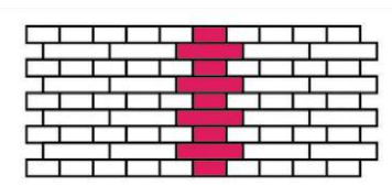
Крестовая кладка
