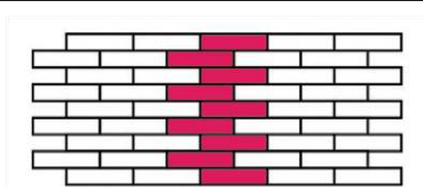
Ложковая кладка
