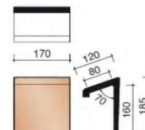
Пультовая моночерепица 70°
