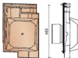
Проходной комплект для вентиляции (D=150мм)
