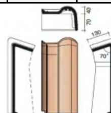
Боковая пультовая моночерепица правая
