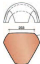
Вальмовая черепица (3 направления)
