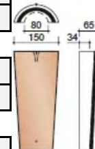
Хребтовая черепица полукруглая
