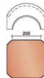
Вальмовая черепица (4 направления)
