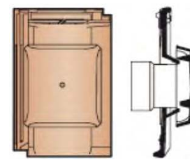
Вентиляционная черепица Проходной комплект для вентиляции (D=150мм)
