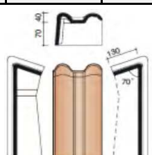
Боковая пультовая моночерепица левая
