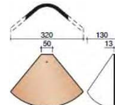
Хребтовая черепица "bonnet grand'mère"
