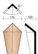
Начальная хребтовая угловая черепица Rustica малая
