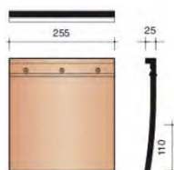
Черепица 3/2
