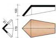
Начальная хребтовая угловая черепица 301 малая
