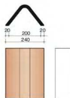
Коньковая угловая черепица Rustica
