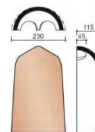
Вальмовая черепица полукруглая
