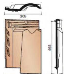
Подконьковая черепица
