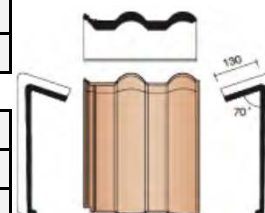
Пультовая моночерепица
