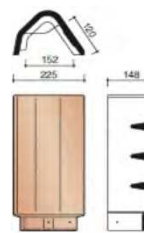
Пультовая черепица
