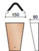
Хребтовая черепица угловая малая
