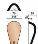
Начальная хребтовая черепица угловая малая
