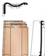
Боковая черепица левая
