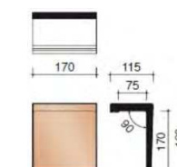
Пультовая моночерепица 90°
