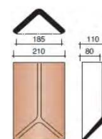
Вальмовая черепица (для хребта bonnet)
