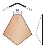
Хребтовая черепица угловая
