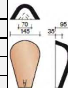
Начальная хребтовая черепица угловая малая
