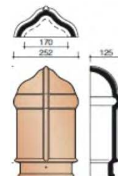
Начальная хребтовая черепица Standard
