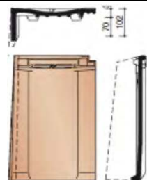
Боковая черепица левая
