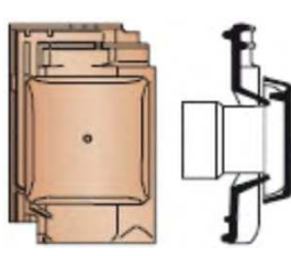
Проходной комплект для вентиляции (D=110мм)
