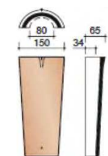
Хребтовая черепица полукруглая
