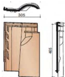
Вентиляционная черепица
