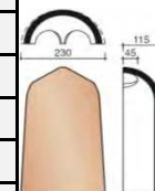
Вальмовая черепица полукруглая
