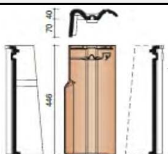
Боковая черепица левая
