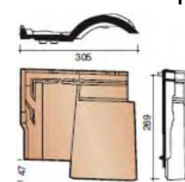
Подконьковая черепица укороченная 3/4
