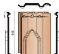
Вентиляционная черепица
