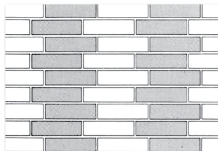
Ложковая перевязка со сдвигом на кирпича по вертикали
