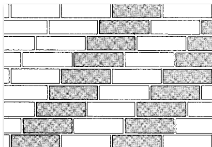
Ложковая перевязка со сдвигом на кирпича по диагонали
